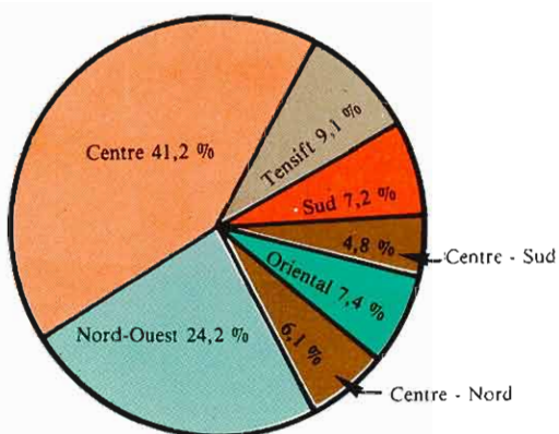
Ventes d'électricité par région économique 1988
